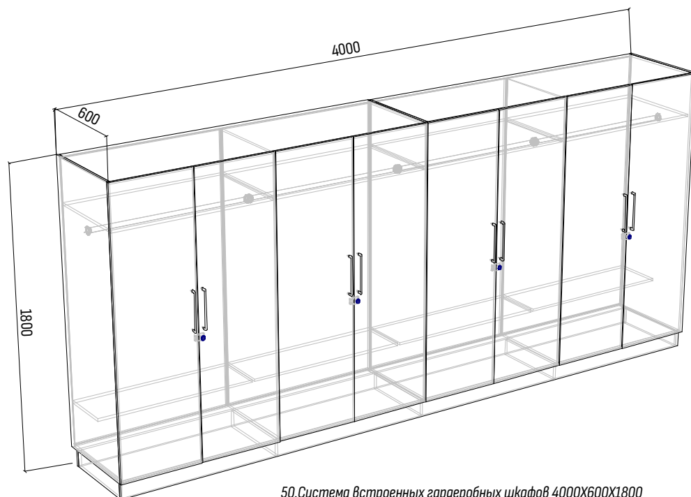
50. Система встроенных гардеробных шкафов 4000X600X1800
